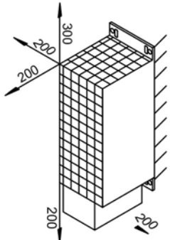
Zulässige Wandmontage Klemmen unten
