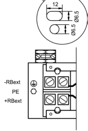
Zulässige Wandmontage Klemmen unten
